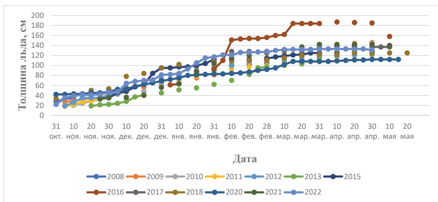
Рис. 4. Сезонный ход нарастания льда за период 2008–2022 гг.
