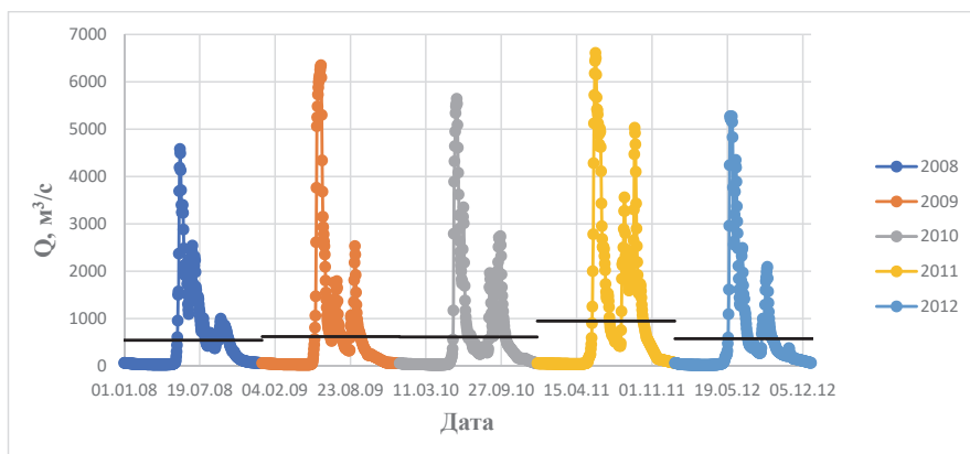
Рис. 1. Ежедневный ход расходов воды р. Пенжина – с. Каменское за 2008–2012 гг.
