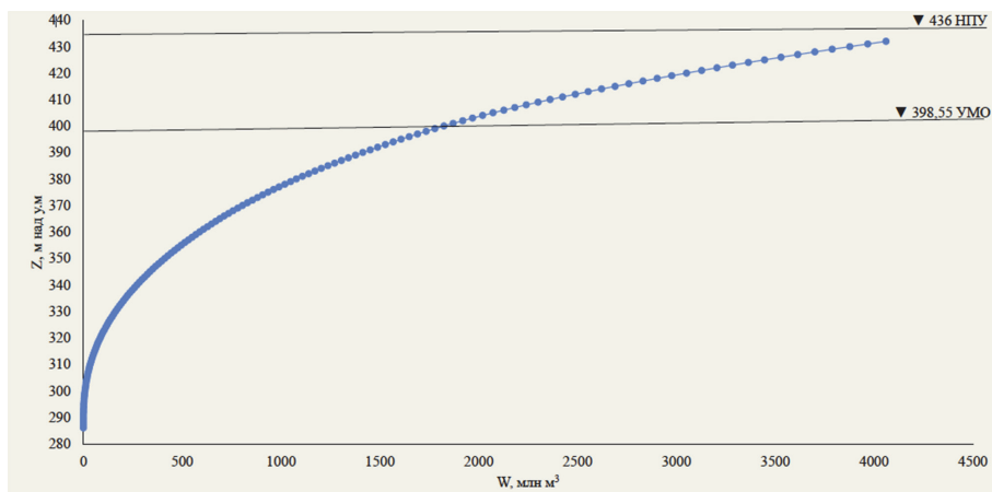
Рис. 2. Кривая связи уровней в верхнем бьефе водохранилища Тельмамской ГЭС и объемов водохранилища
