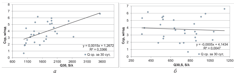
Рис. 2. График зависимости средних скоростей размыва ( C_{cp} , м):
