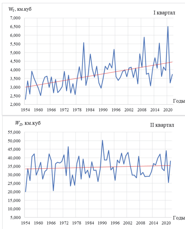
Рис. 1. Многолетнее (1954–2022 гг.) изменение притока воды к Камскому водохранилищу за I–II квартал
