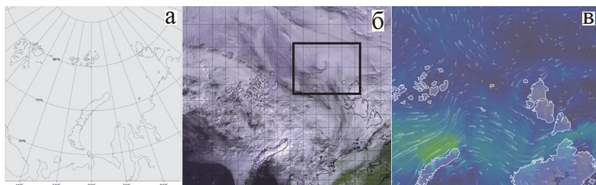
Рис. 3. Прогностическая карта испытательного полигона от 0 часов UTC 8 августа 2024 г. (а), спутниковое изображение той же области с сайта Метео-Сибирь от 5:30 UTC 8 августа 2024 г. с распределением облачности в виде завихрения с координатами центра 82° с. ш. 82° в. д. (б) и поле приземного ветра на 6:00 UTC 8 августа 2024 г., рассчитанное по модели GFS с сайта https://www.ventusky.com (в)
