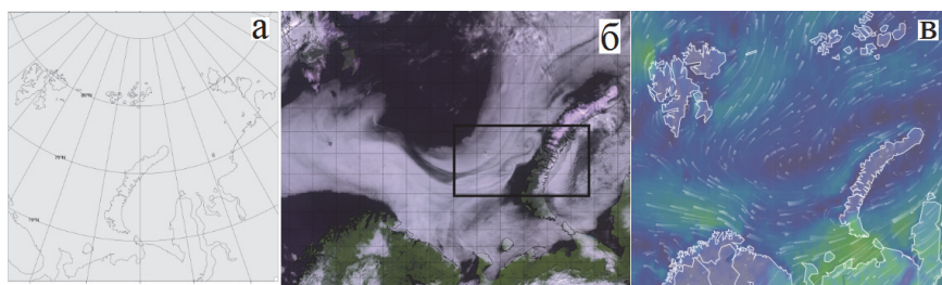
Рис. 2. Прогностическая карта испытательного полигона от 0 часов UTC 4 августа 2024 г. (а), спутниковое изображение той же области с сайта Метео-Сибирь от 7:45 UTC 4 августа 2024 г. с распределением облачности в виде завихрения с координатами центра 74° с. ш. 52° в. д. (б) и поле приземного ветра на 6:00 UTC 4 августа 2024 г., рассчитанное по модели GFS с сайта https://www.ventusky.com (в)
