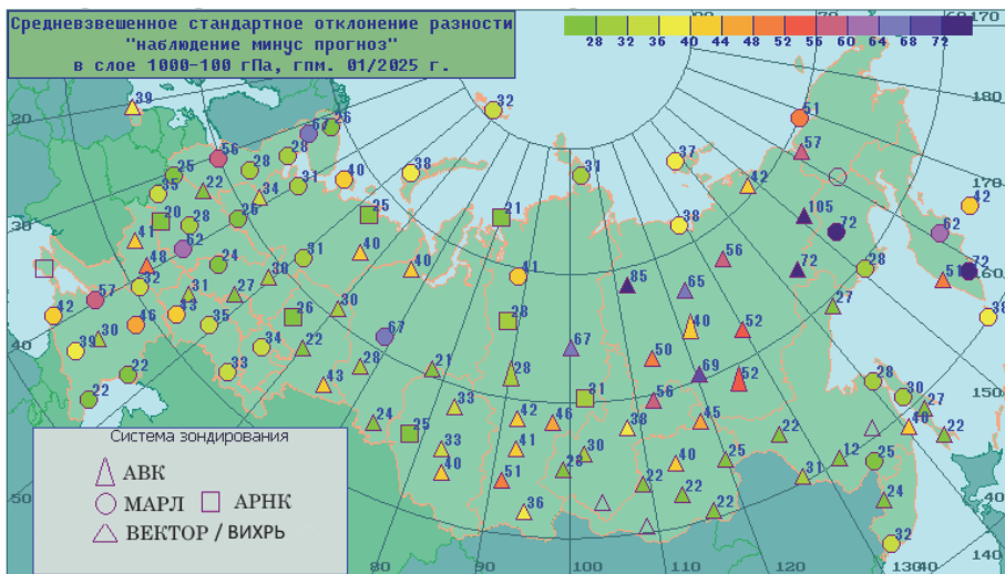
Рис. Взвешенное среднеквадратичное значение 'наблюдение-прогноз' для геопотенциала в слое 1000–100 гПа в январе 2025 г.
