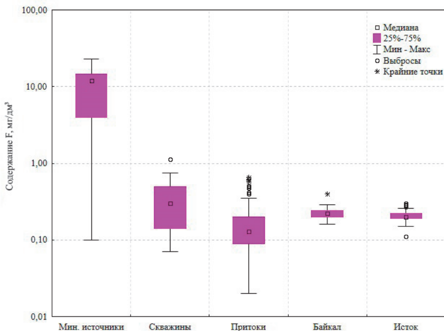
Рис. 3. Распределение концентраций F в сопряженных водных компонентах экосистемы Байкала (мг/дм³)
