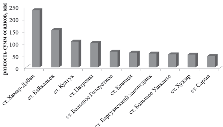
Рис. 2. Годовая амплитуда атмосферных осадков на прибайкальских станциях Иркутской области за период 1980–2023 гг.
