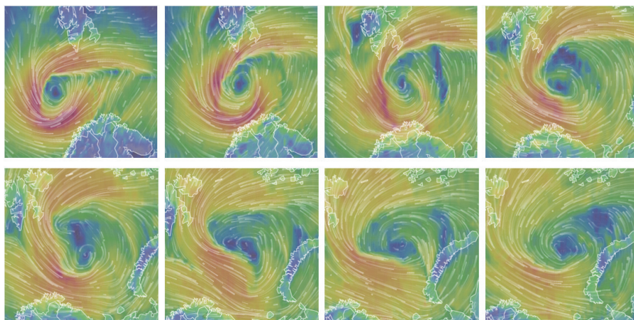
Рис. 6. Поля приземного ветра, рассчитанные по модели GFS с сайта https://www.ventusky.com за период с 0 ч UTC 29.11.2024 по 18 ч UTC 30.11.2024 с шагом 6 ч
