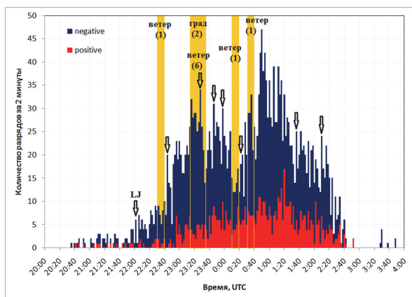
Рис. 3. Динамика во времени количества молниевых разрядов для мощного шторма, прошедшего по западу ЕТР 18–19.05.2021 г. с указанием случаев выявления сигнатуры LJ и моментов регистрации различных ОКЯ
