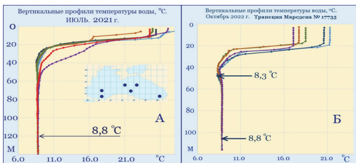
Рис. 1. Вертикальные профили температуры воды (измерения буем АРГО)
