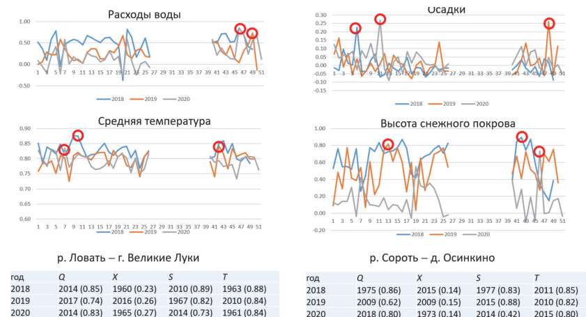
Рис. 2. Годовая корреляция
