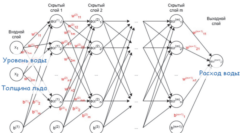
Рис. 5. Схематическое изображение модели нейронной сети прямого распространения для связи уровня воды и толщины льда с расходом воды.
