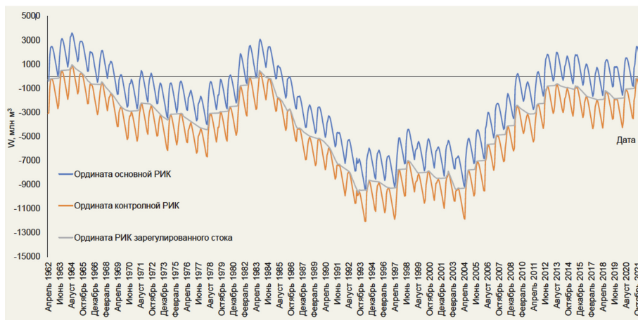
Рис. 3. Разностно-интегральные кривые
