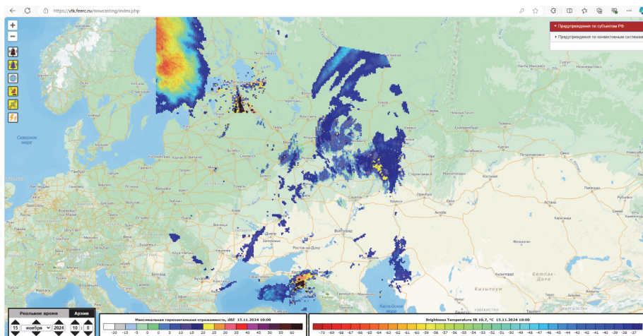
Рис. 5. Веб-ГИС прототипа технологии
