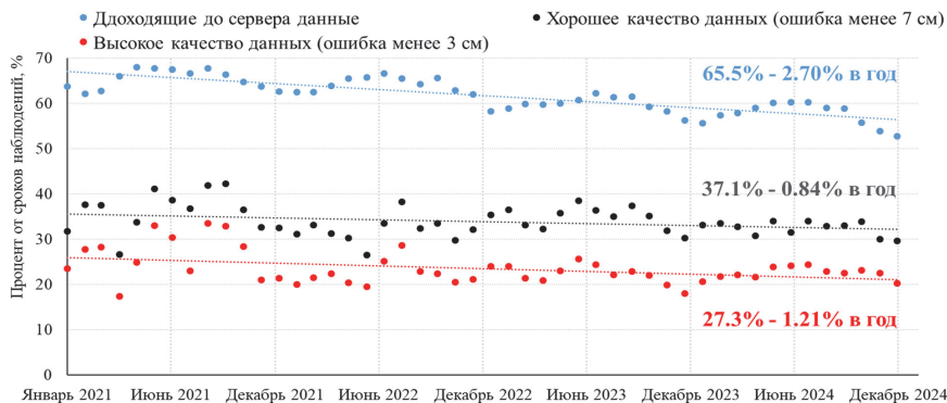
Рис. 3. Динамика работы АГК за 2021–2024 гг.
