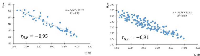
Рис. 4. График связи площади о. Ярки и фактических уровней оз. Байкал (слева) и График связи площади о. Ярки и расчетных уровней оз. Байкал (справа)
