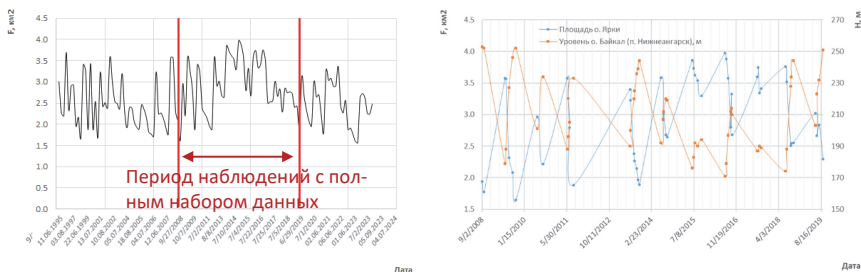
Рис. 3. Результат работы алгоритма – рассчитанные площади о. Ярки (слева) и График изменения площади о. Ярки и уровней оз. Байкал (справа)
