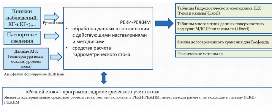
Рис. 1. Схема обработки гидрологических данных и формирование продукции системой РЕКИ-РЕЖИМ
