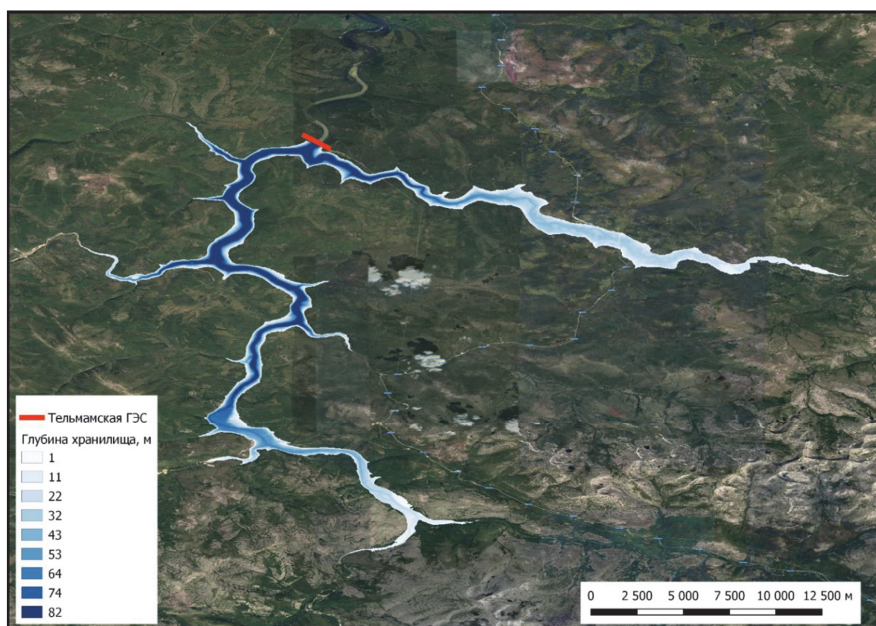
Рис. 1. Створ размещения (красная линия) и зона затопления проектируемым водохранилищем Тельмамской ГЭС
