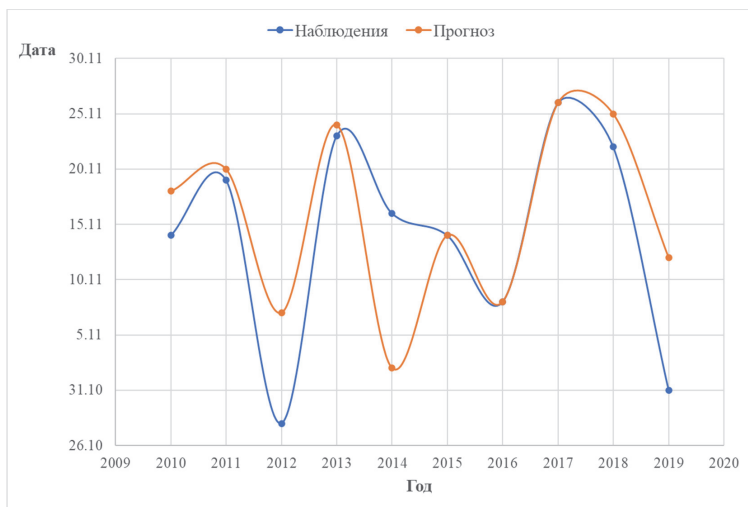
Рис. 3. Прогноз дат установления ледостава на р. Умба – порог Паялка
