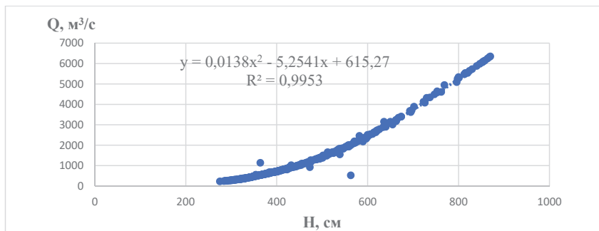
Рис. 6. Кривая Q(H) для свободного русла за период 2008–2010 гг.
