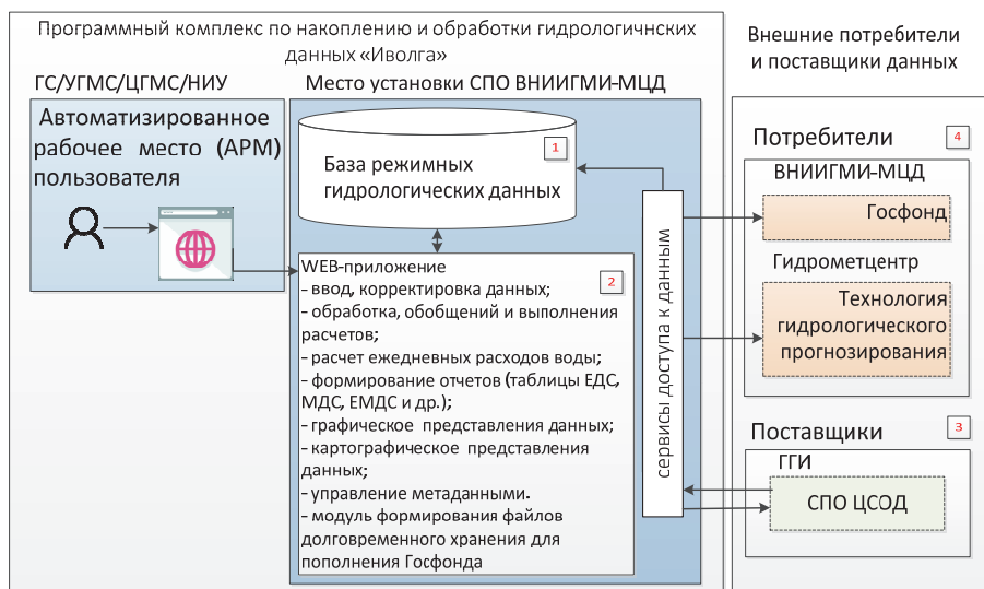
Рис. 3. Архитектура и компоненты новой системы обработки гидрологических данных: 1 – центральное хранилище гидрологических данных и продукции; 2 – сервер приложений, содержит весь необходимый функционал для работы с гидрологическими данными и средства подготовки продукции; 3 – системы сбора данных, которые являются поставщиками данных, поступающих по автоматизированным каналам связи; 4 – внешние системы, которые являются потребителями гидрологических данных, доступ к центральной БД осуществляется посредством web-сервисов
