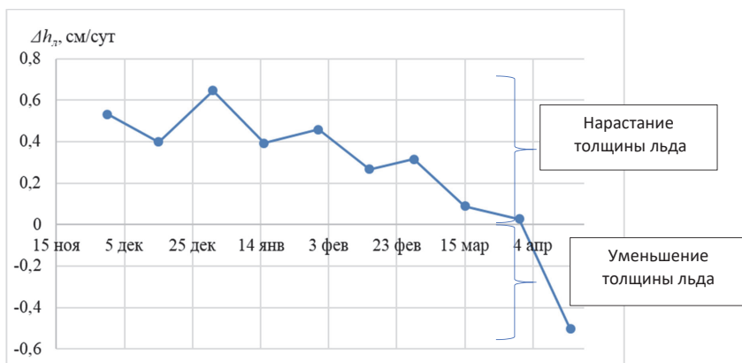
Рис. 2. Среднее по всем г/п Камского водохранилища изменение интенсивности нарастания толщины льда ( \Delta h_{\text{л}} , см/сут) за период 1956–2023 гг.
