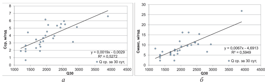
Рис. 1. График зависимости средних (а) и максимальных (б) скоростей размыва ( C_{\text{ср}} и C_{\text{макс}} , м) от расхода, который был превышен 30 дней в году ( Q_{30} , м 3 /с)
