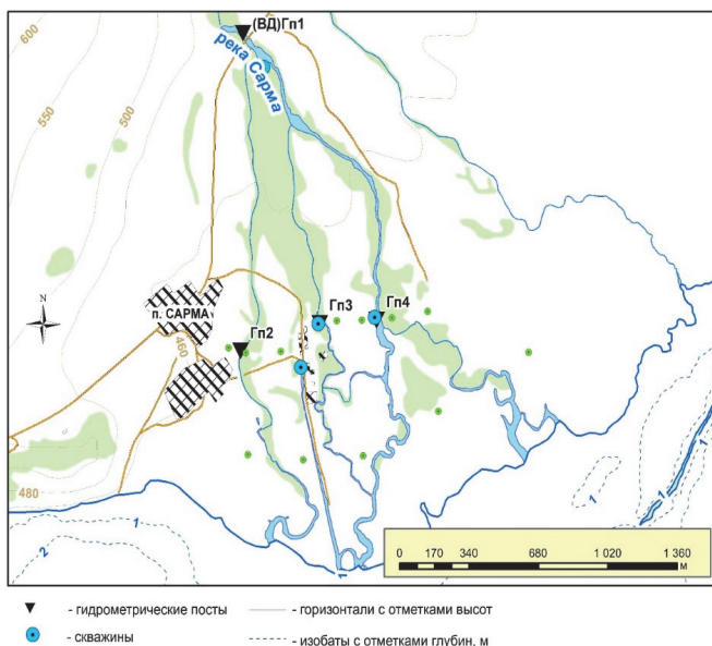
Рис. 1. Расположение гидрологических створов и скважин в УС Сарма
