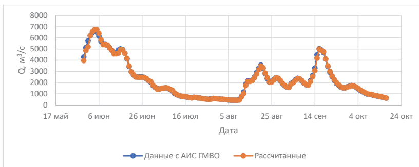
Рис. 7. Ежедневные расходы воды за период свободного русла, взятые из АИС ГМВО и рассчитанные по уравнению линейной регрессии за 2011 год
