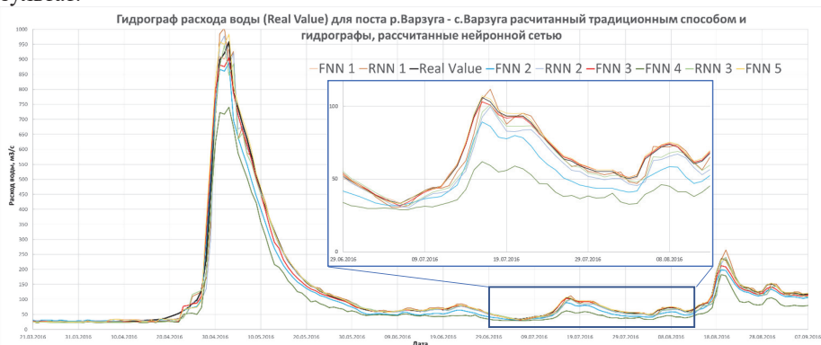
Рис. 6. Гидрограф расхода воды для поста р. Варзуга – с. Варзуга рассчитанный традиционным способом и гидрографы, рассчитанные нейронной сетью.
