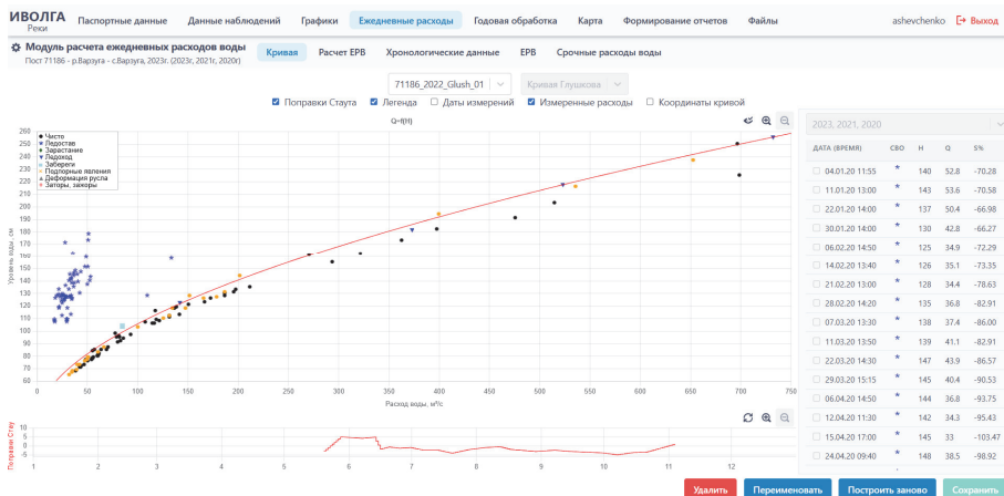
Рис. 4. Модуль расчета ежедневных расходов воды в системе «Иволга». Автоматический подбор кривой зависимости Q(H)
