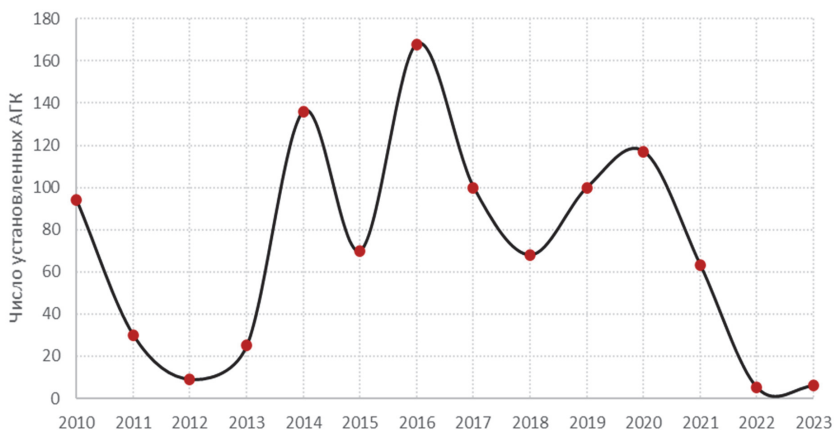
Рис. 1. Распределение по годам количества введённых в эксплуатацию АГК
