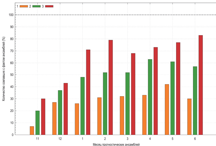
Рис. 2. Количество ансамблей с точностью прогнозирования относительного фактического показателя: 1 – 0,5°C, 2 – 1°C, 3 – 1,5°C
