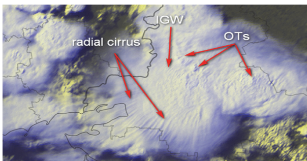
Рис. 2. Спутниковые сигнатуры градового шторма в Ростовской области 14.06.2020. (Meteosat, видимый диапазон)
