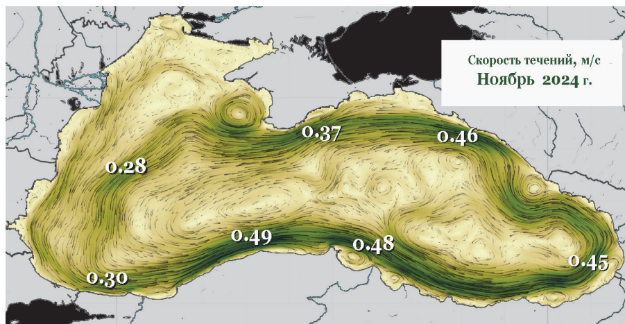
Рис. 4. Карта поверхностных течений Черного моря по модельным расчетам (расчет выполнен в рамках проекта Коперникус)
