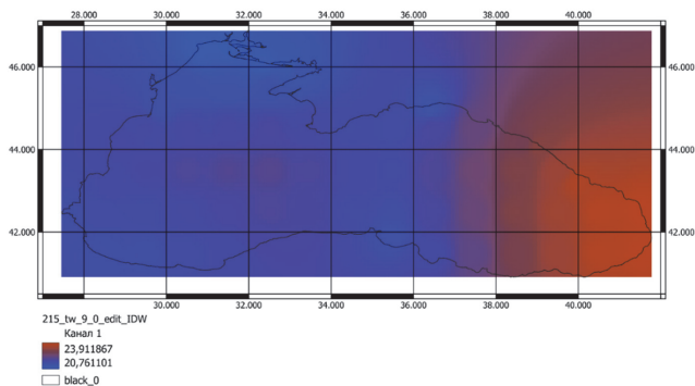
Рис. 1. Интерполяция: ОВР
