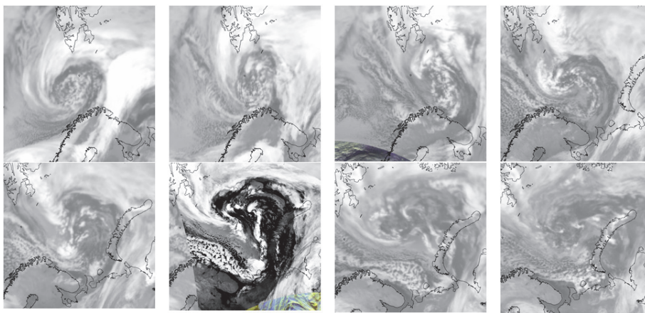
Рис. 4. Спутниковые изображения с ПМЦ (Арктика-М № 1 и № 2, NOAA-18 и 19) за период с 0 ч UTC 29.11.2024 г. по 18 ч UTC 30.11.2024 г. с шагом 6 ч
