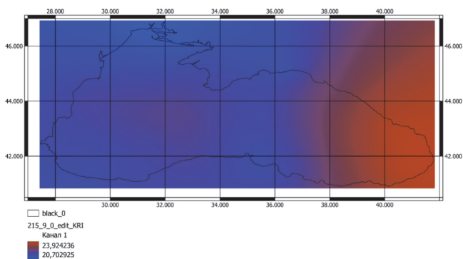
Рис. 2. Интерполяция: кригинг
