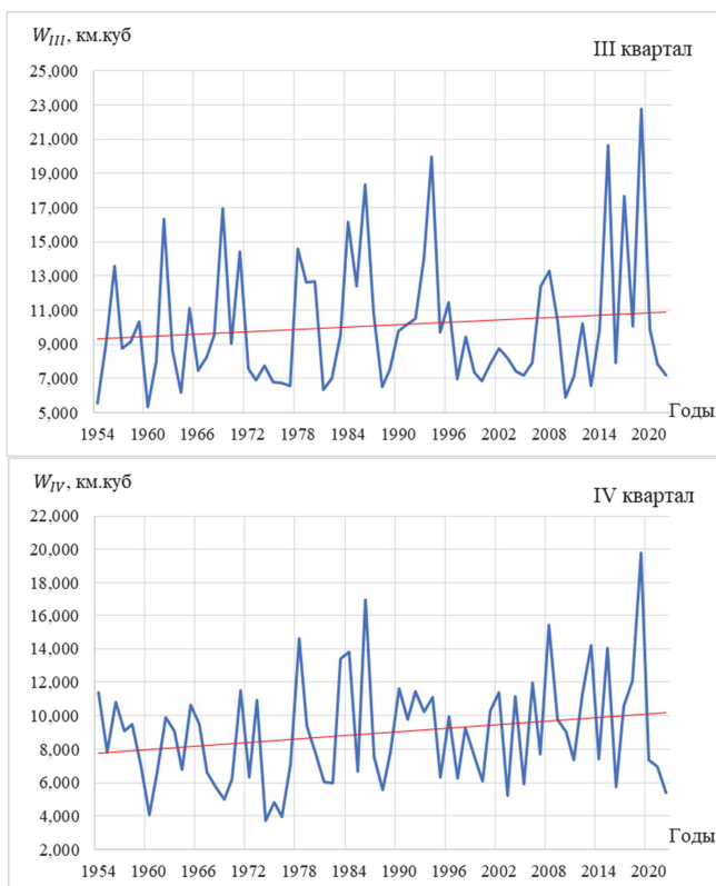
Рис. 2. Многолетнее (1954–2022 гг.) изменение притока воды к Камскому водохранилищу за III-IV квартал
