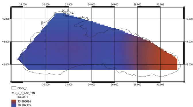
Рис. 3. Интерполяция: триангуляция
