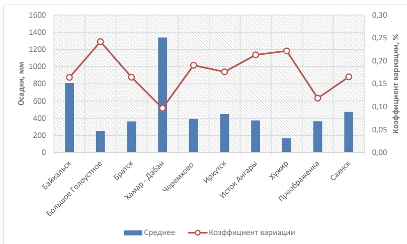
Рис. 2. Среднеголетняя годовая сумма осадков и коэффициент вариации данных станций ХСО Иркутской области за период с 2010 по 2020 г.
