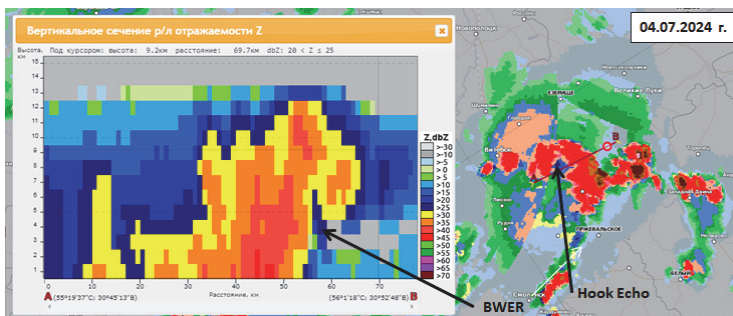
Рис. 1. Радарные сигнатуры суперячейки, прошедшей по территории северо-западного федерального округа 4 июля 2024 г. (веб-ГИС «Метеорад»)
