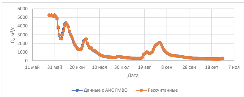
Рис. 8. Ежедневные расходы воды за период свободного русла, взятые из АИС ГМВО и рассчитанные по уравнению линейной регрессии за 2012 год
