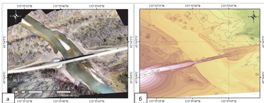
Рис. 2. Ортофотоплан (а) и карта высот (б) нижнего течения р. Извилинка СК WGS-84
